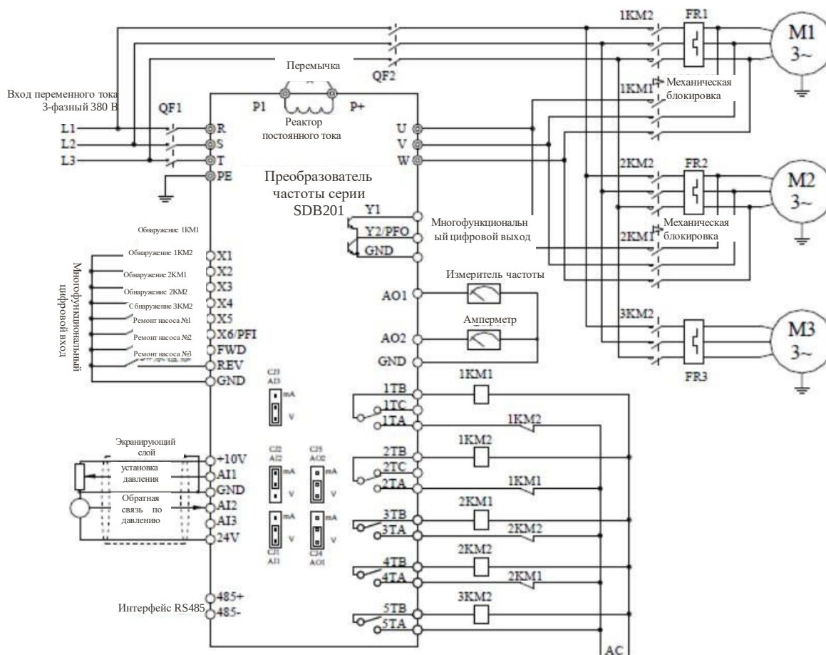
Схема применения включения по циклу частотного преобразования "один управляет два" и вспомогательного насоса
