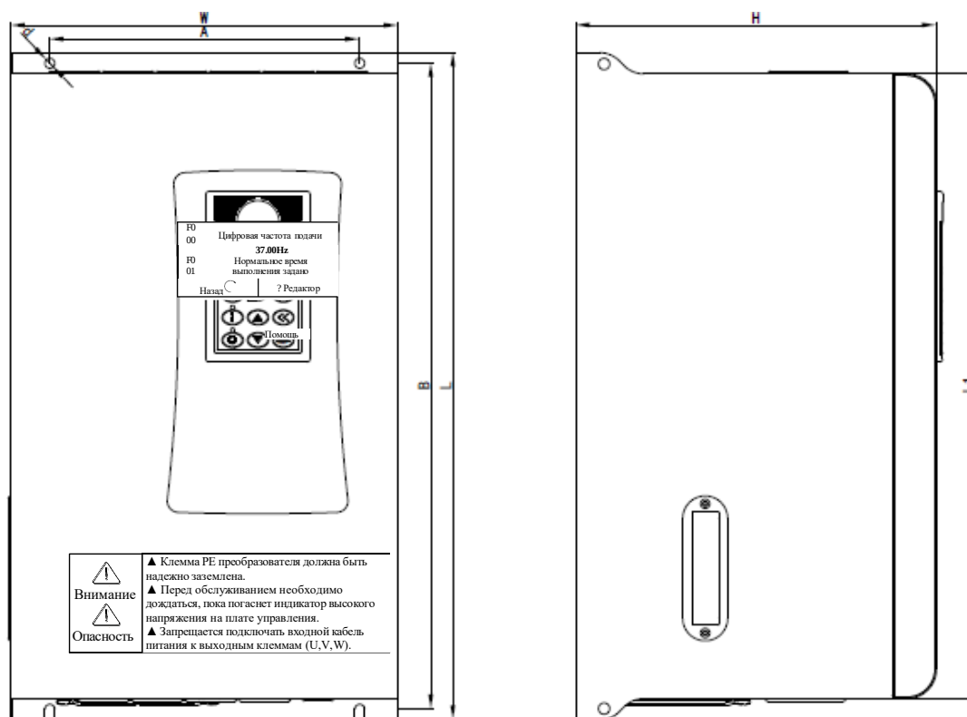
Эскизный чертеж модели SDB201-030K/04 и выше
