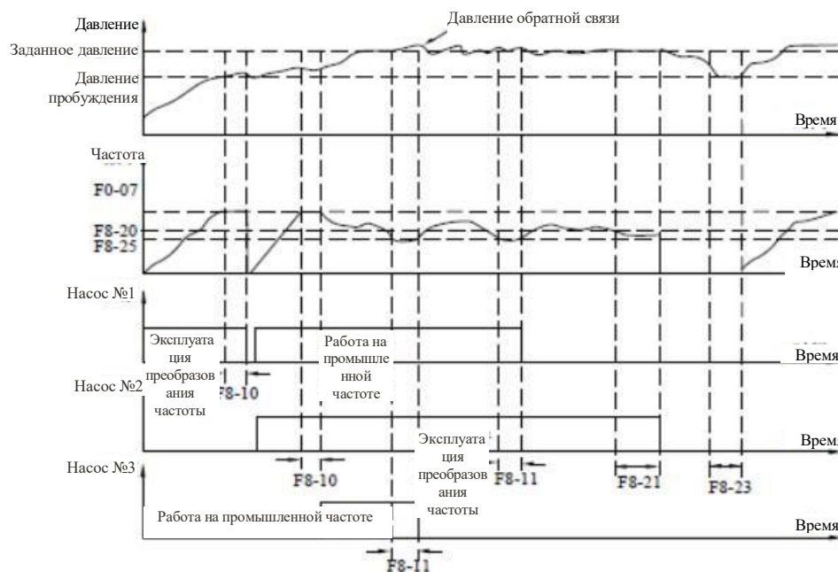
Временная диаграмма работы системы
