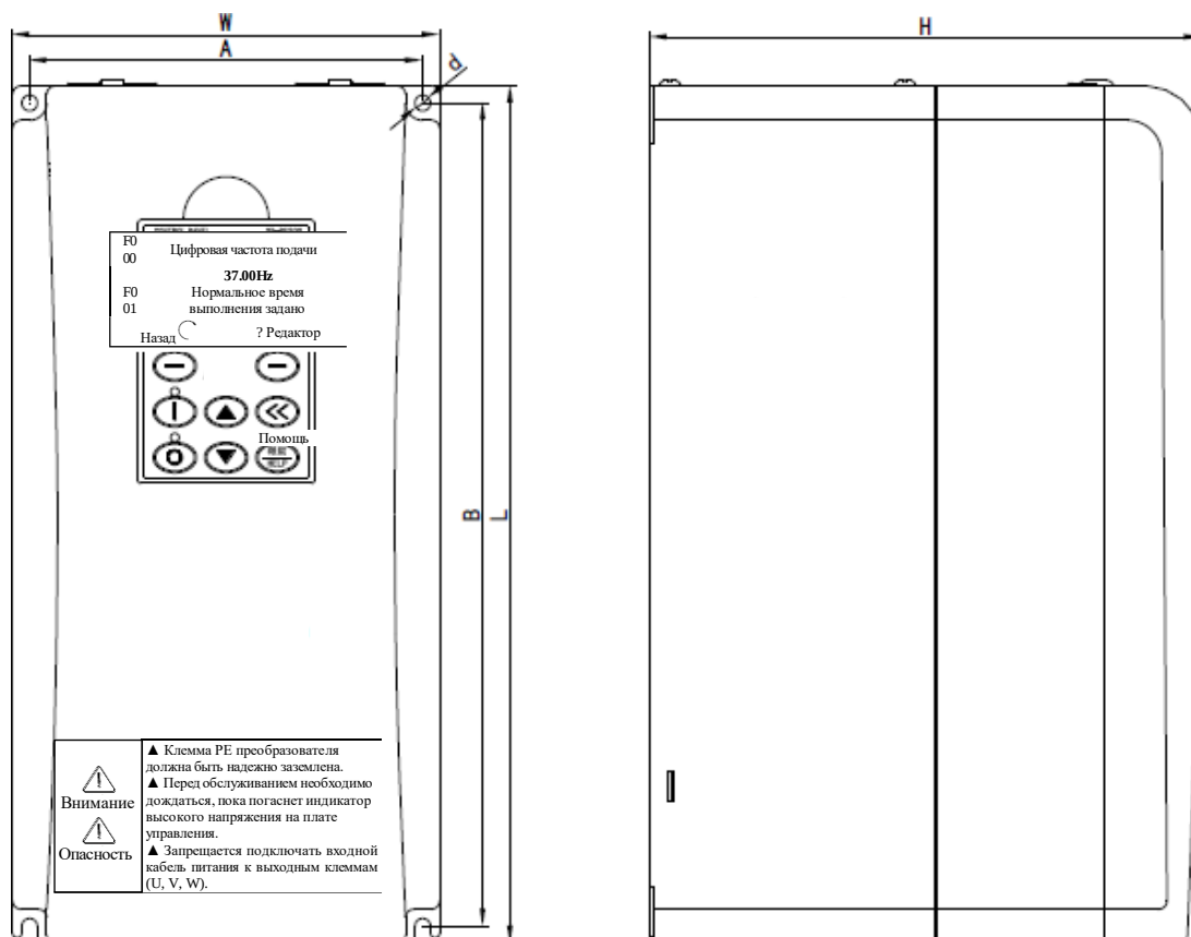
Эскизный чертеж модели SDB201-07K5/04~ 022K/04
