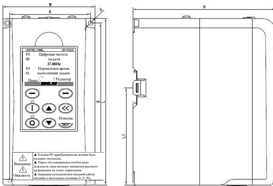
Чертеж модели SDB201-01K5/04~:05K5/04(поставляется для стандартного монтажа на DIN-рейку)
