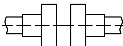
Рис. 2.5.2. Параллельная несоосность
