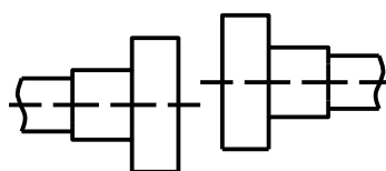
Рис. 2.5.2. Параллельная несоосность
