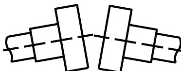
Рис. 2.5.1. Угловая несоосность
