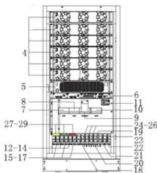
Вид спереди на внутреннюю часть шкафа
